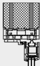
Verbreiterungselement
